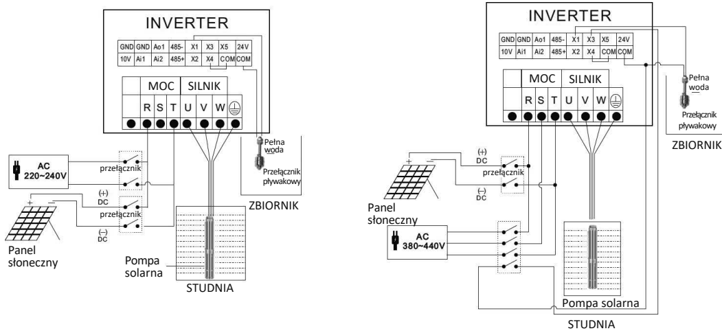
Rysunek instalacji systemu
