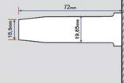
ΣΧΕΔΙΟ 6 ΣΦΗΝΑ 20mm ΓΙΑ ΜΕΙΩΤΗΡΑ
