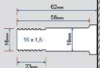
ΣΧΕΔΙΟ 2 ΠΑΙΣΙΟ 19mm (6.5Hp)
